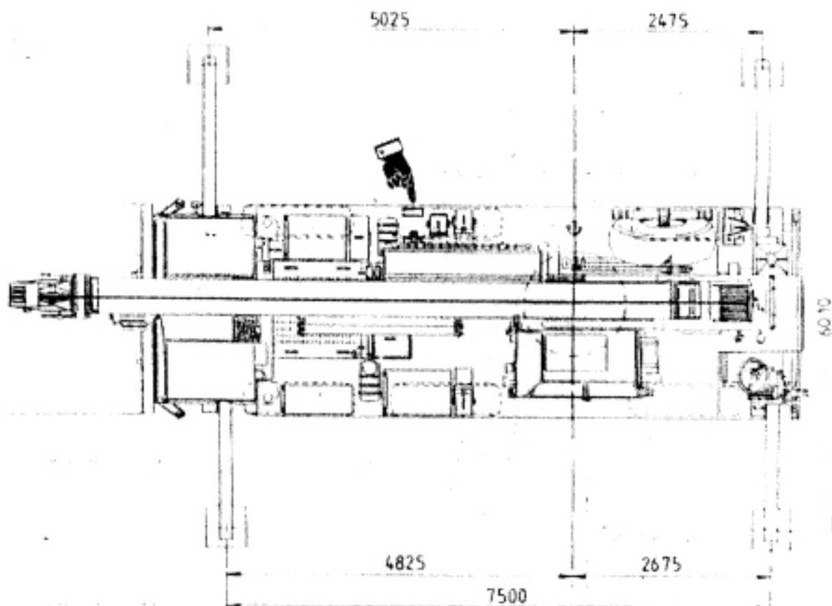
Rys. 6 Wymiary w pozycji gotowej do transportu i rozłożonych podporach
